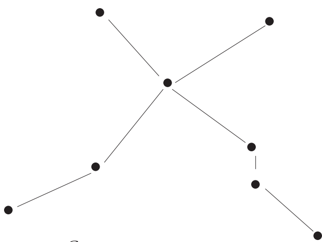
Cygnus
